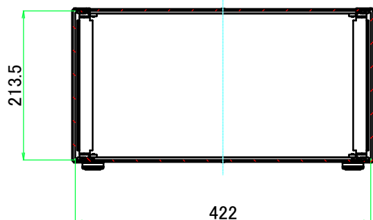
A-A ( 1 : 7.5 )
